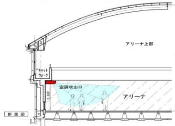
空調設備設置イメージ図②
