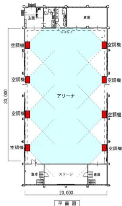
空調設備設置イメージ図①
