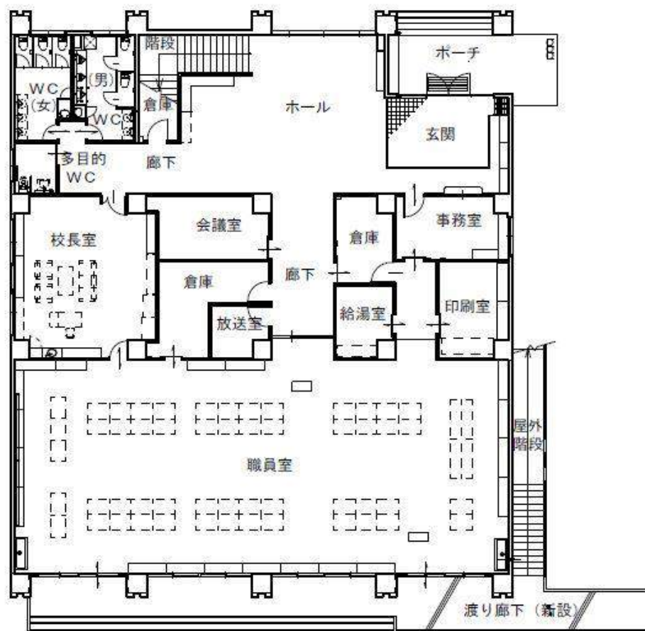
1 階 平 面 図
