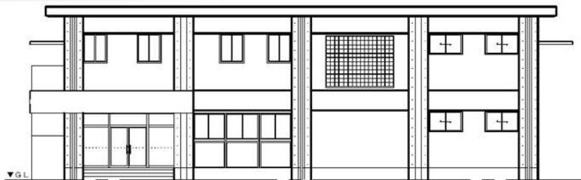
北側立面図
